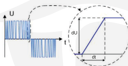
Напряжение на обмотках двигателя с dU/dt дросселем
