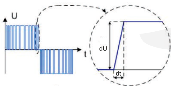
Напряжение на обмотках двигателя без dU/dt дросселя
