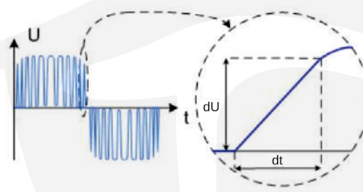
Напряжение на обмотках двигателя с моторным дросселем
