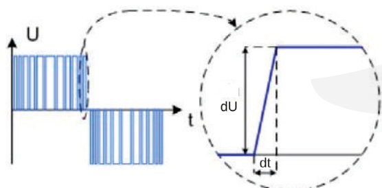
Напряжение на обмотках двигателя без моторного дросселя
