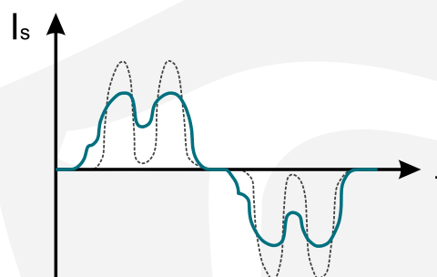
Входной ток преобразователя частоты с сетевым дросселем
