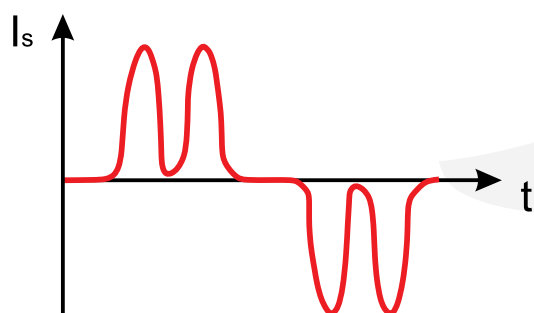
Входной ток преобразователя частоты без сетевого дросселя
